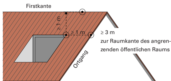
Beispiel Satteldach
