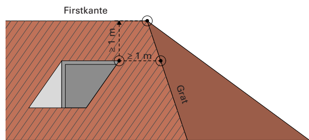
Beispiel Walmdach
