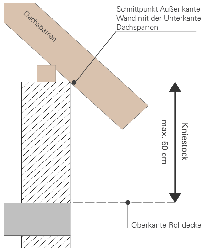
Zeichnerische Begriffserläuterung zum Kniestock
